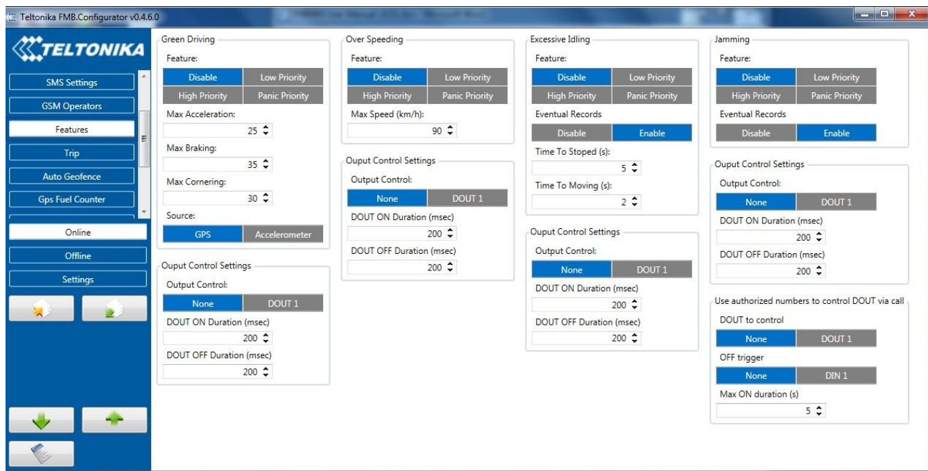
Рис.18 Настройка сценариев
