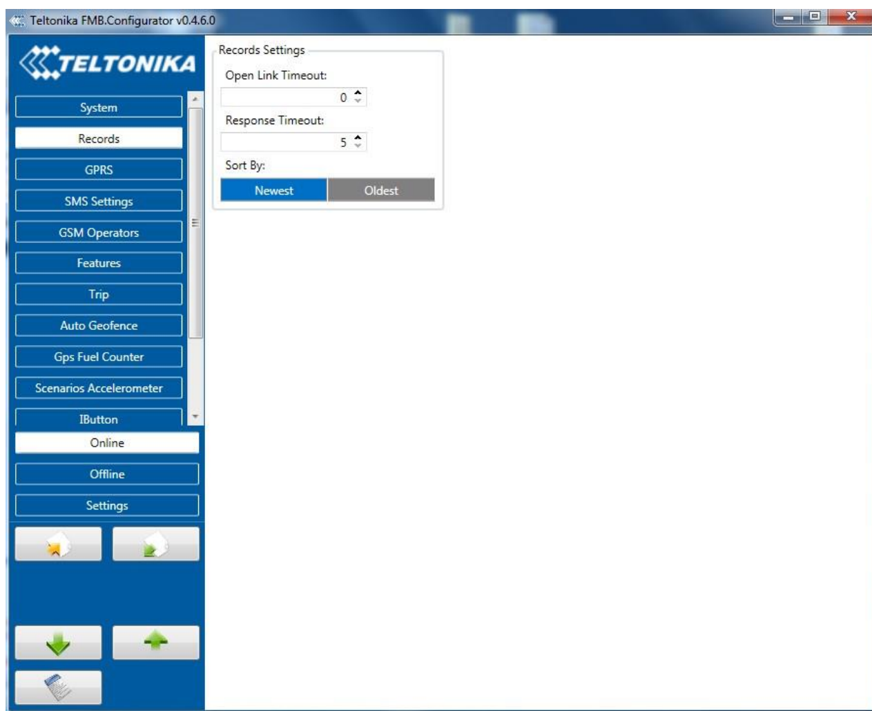
Рис. 12 Конфигурация записей
