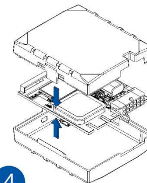
Рисунок 7 Установка крышки на место
