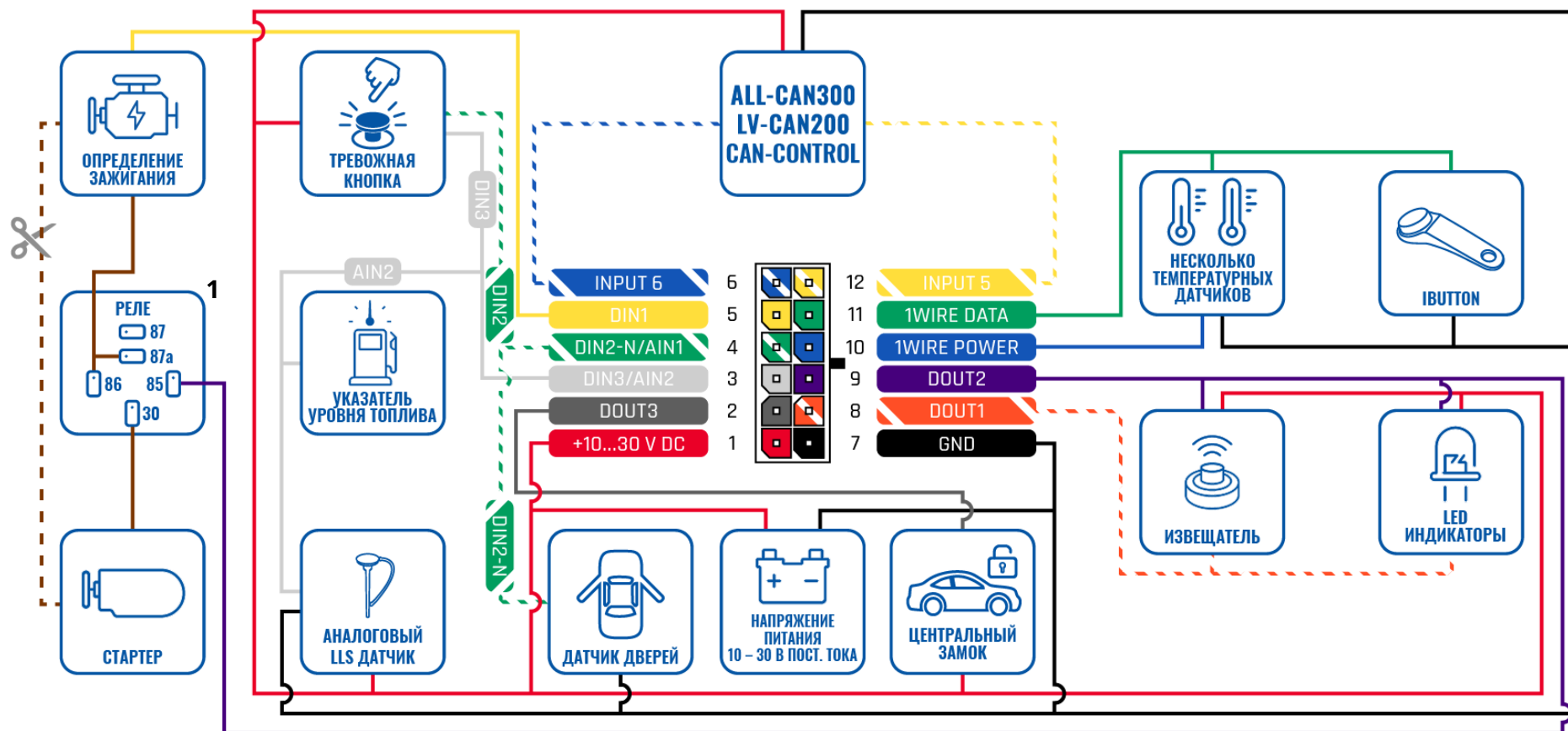
Рисунок 2 FMC130 Схема подключения
