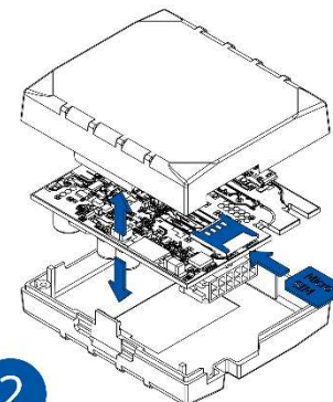
Рисунок 5 Вставка Micro-SIM карты
